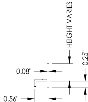
60 SILL RISER
