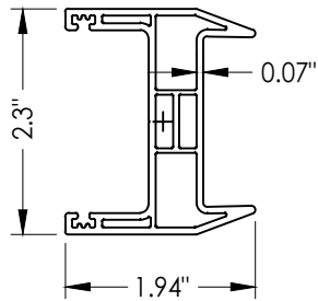
11 ASTRAGAL
